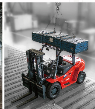
护顶架冲击试验
