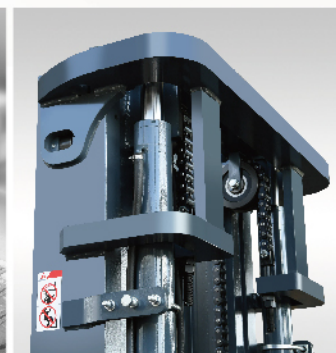
框架式上横梁结构，受力更合理，提升刚度和强度
